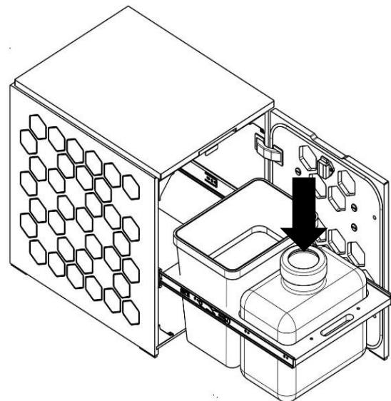
Urinkanister einsetzen
