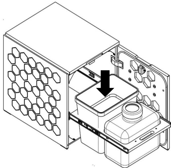
Feststoffbehälter einsetzen
